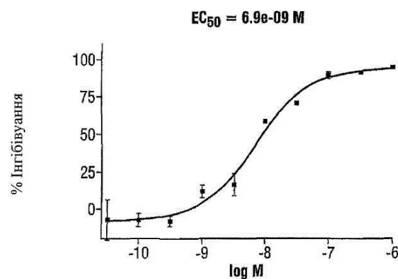
ФІГ. 4 (СПОЛУКА 67)
