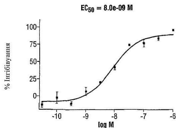
ФІГ. 2 (СПОЛУКА 48)
