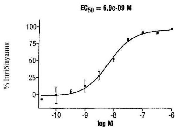
ФІГ. 1 (СПОЛУКА 7)
