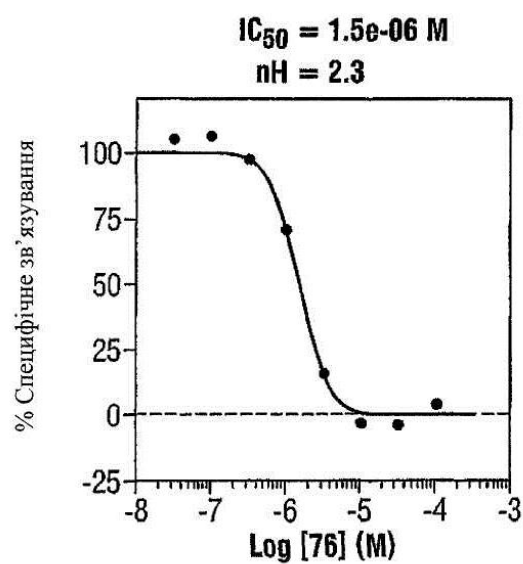
ФІГ. 11 (Крива конкуренції для сполуки 76 на рецепторі NK2 людини)
