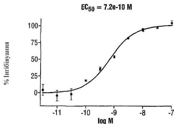
ФІГ. 3 (СПОЛУКА 66)
